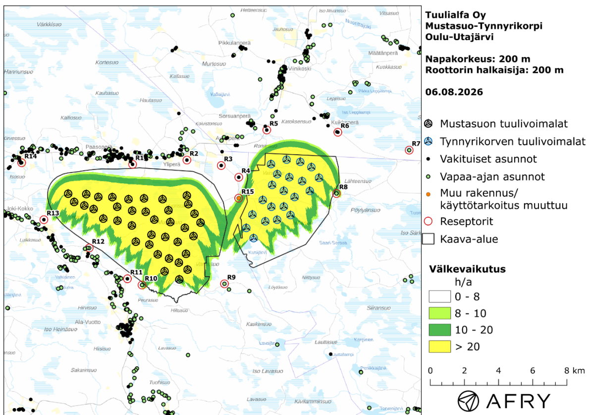
Kuva 3-3: Mustasuo-Tynnyrikorven voimaloiden todennäköinen vuotuinen välkevaikutus.
