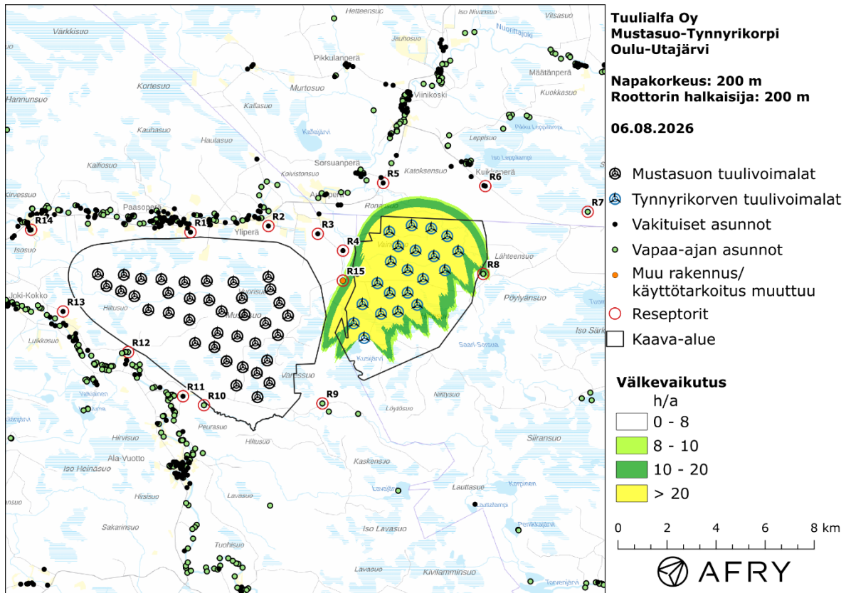
Kuva 3-2: Tynnyrikorven voimaloiden todennäköinen vuotuinen välkevaikutus.
