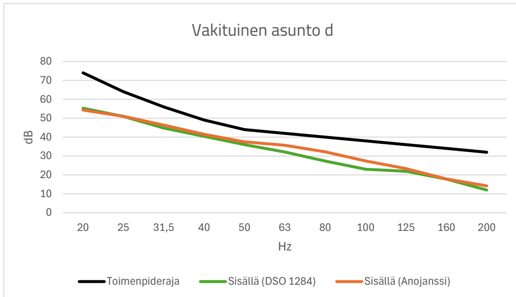
Kuva 3. Ympäristöministeriön ohjeistuksen mukainen pienitaajuisen melun laskenta sekä sosiaali- ja terveysministeriön toimenpiderajat vakituksessa asunnossa d.
