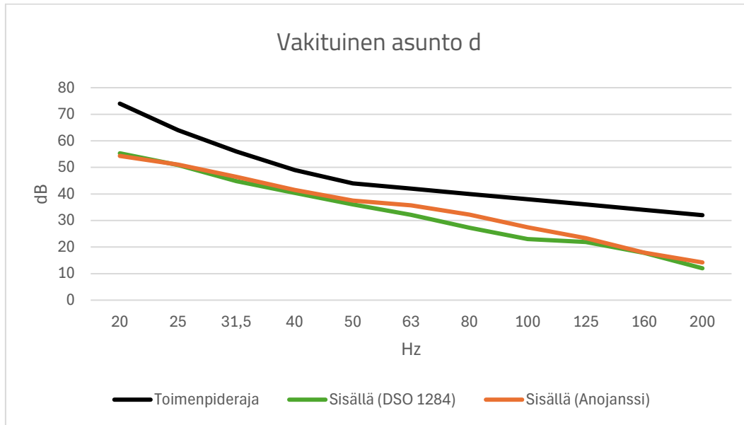
Kuva 5. Ympäristöministeriön ohjeistuksen mukainen pienitaajuisen melun laskenta sekä sosiaali- ja terveysministeriön toimenpiderajat vakituisesa asunnossa d.
