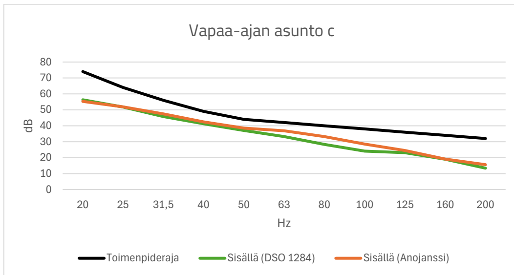
Kuva 4. Ympäristöministeriön ohjeistuksen mukainen pienitaajuisen melun laskenta sekä sosiaali- ja terveysministeriön toimenpiderajat vapaa-ajan asunnossa c.
