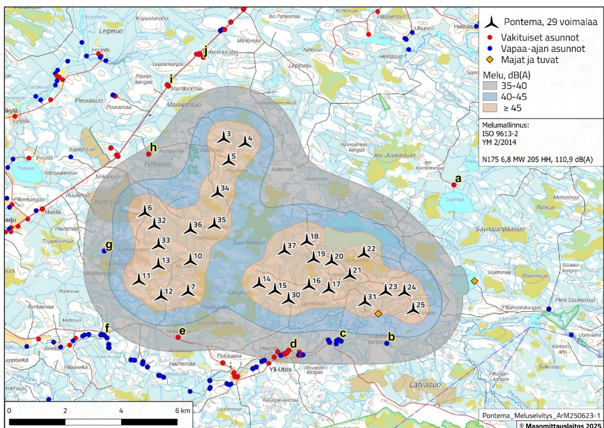
Kuva 1. Ponteman tuulivoimapuiston melumallinnus, N175 6,8 MW 205 m HH 110,9 dB(A). Kymmenen havainnointipistettä on merkitty kuvaan kirjaimilla.
