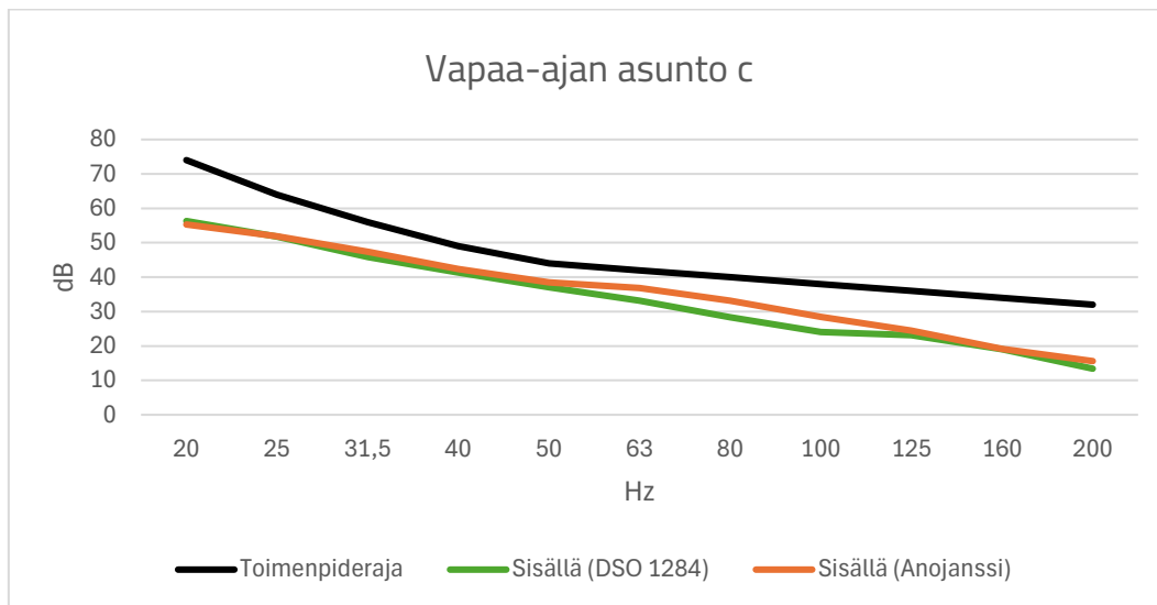
Kuva 6. Ympäristöministeriön ohjeistuksen mukainen pienitaajuisen melun laskenta sekä sosiaali- ja terveysministeriön toimenpiderajat vapaa-ajan asunnossa c.
