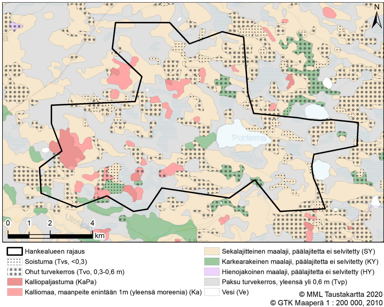
Kuva 4. Hankealueen maaperäkarta.
