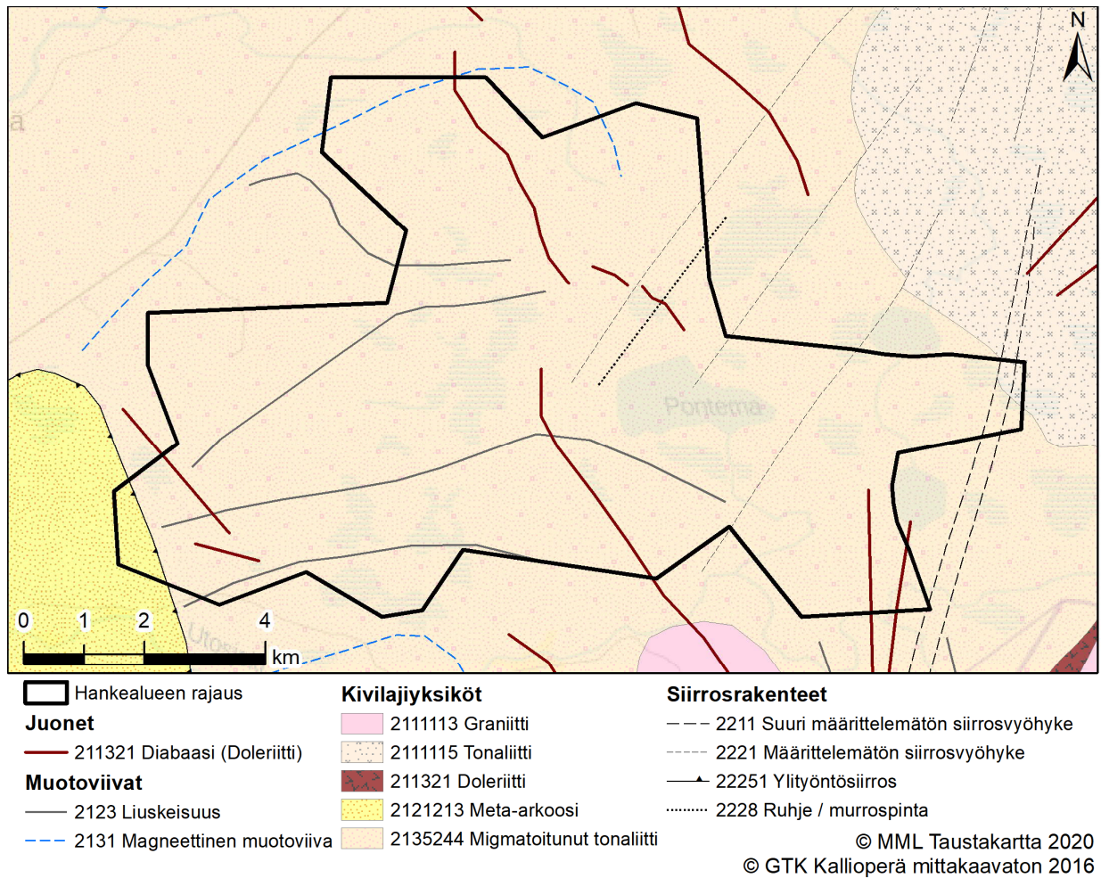
Kuva 3. Hankealueen kallioperäkartta.
