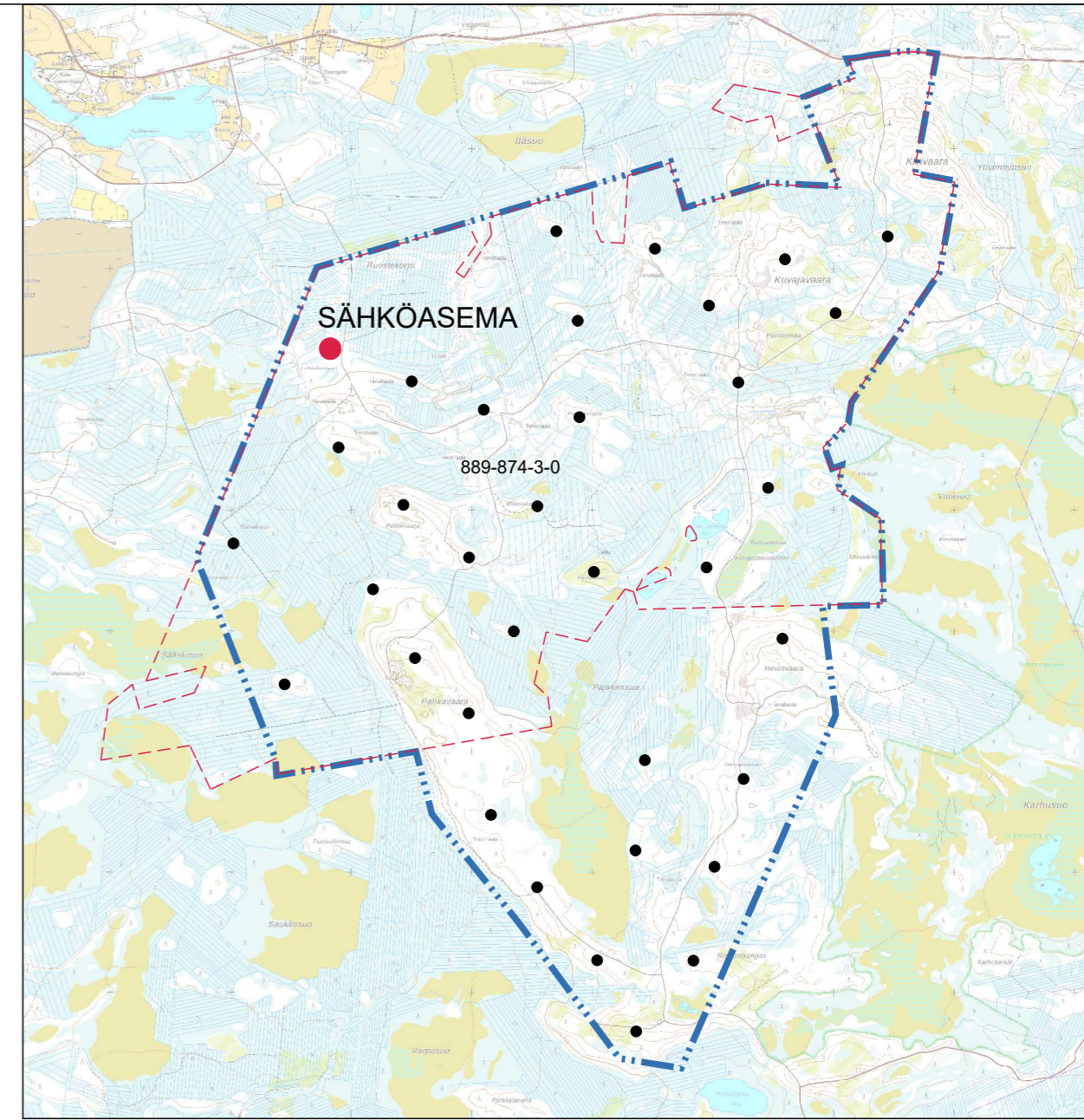
Ohjeellinen sähköasematontti (n.120m*145m aidattu alue). Sähköaseman lopullinen sijoittelu saattaa vielä tarkentua.
